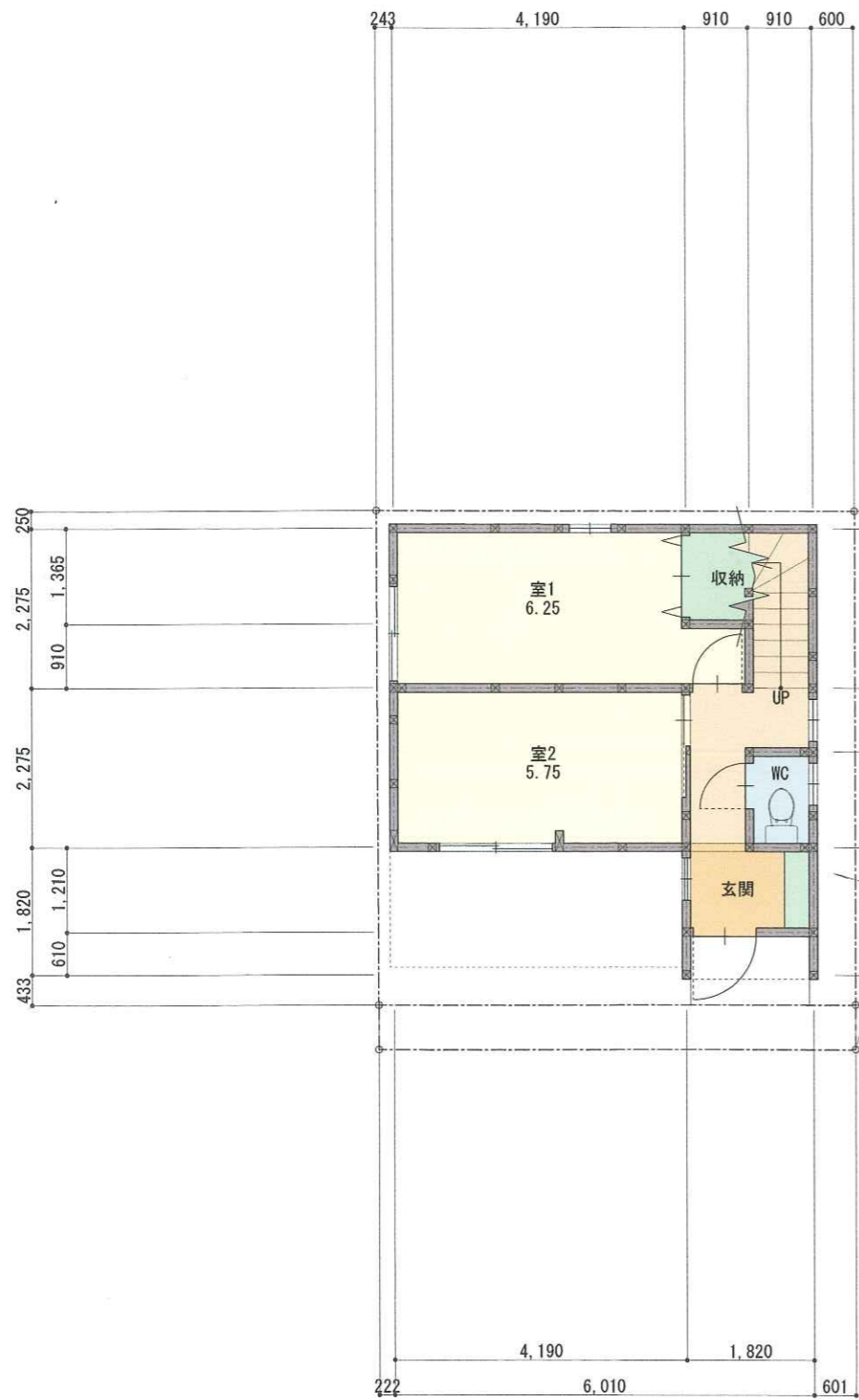
1階平面図
